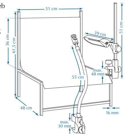
Kaiser Flächenlichtquelle zur Durchleuchtung oder zum Freistellen. backlite 6000 (5463) für Art.-Nr. 5928/29 prolite basic 2 HF (2425) für Art.-Nr. 5997/98
